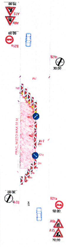
SCHEMA Č. 2 PRACOVNÍ MÍSTO V KOMUNIKACI V INTRAVILÁNU
